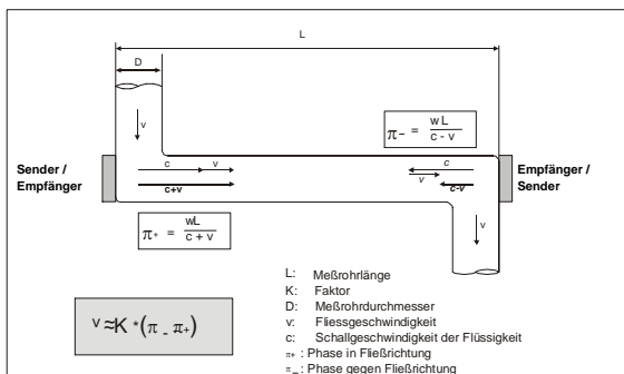
Abb. 1: Prinzipdarstellung der Ultraschalldurchflussmessung
